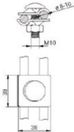
Univerzális csatlakozó tűzi horganyzott acél (StZn), 38 × 38 mm, 1 db M10 × 30-as csavar Köracél keresztmetszete: 8-10 mm
