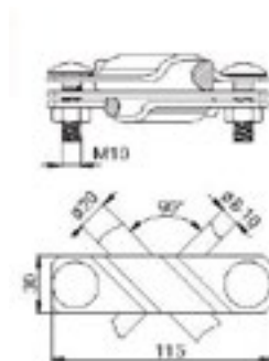
Átlós keresztkapocs tűzi horganyzott acél (StZn), 115 × 30 mm, 2 db M10 × 30-as csavar Köracél keresztmetszete: 8-10 mm
