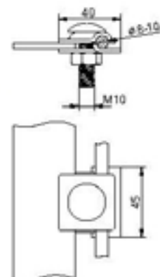
Multikapocs tűzi horganyzott acél (StZn), 45 × 40 mm, 1 db M10 × 30-as csavar Köracél keresztmetszete: 8-10 mm Betételemez mérete: < 5 mm
