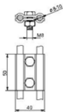
Párhuzamos összekötő tűzi horganyzott acél (StZn), 50 × 40 mm, 2 db M8 × 20-as csavar Köracél keresztmetszete: 8-10 mm
