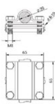
L-65 keresztösszekötő tűzi horganyzott acél (StZn), 65 × 65 mm, 4 db M8 × 25-ös csavar Köracél keresztmetszete: 8-10 mm
