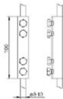
Összekötő kapocs tűzi horganyzott acél (StZn), 100 mm, 4 db M6 × 10-es csavar Köracél keresztmetszete: 8-10 mm
