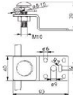
Csatlakozóidom csatlakozó-kapoccsal tűzi horganyzott acél (StZn), 90 × 40 × 38 mm, 1 db M10 × 30-as csavar Köracél keresztmetszete: 8-10 mm
