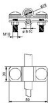
Leválasztó kapocs tűzi horganyzott acél (StZn), 80 × 30 mm, 2 db M10 × 30-as csavar Köracél keresztmetszete: 8-10 mm
