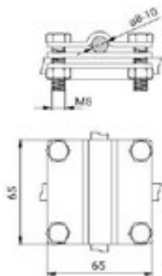
L-65 Keresztösszekötő csatlakozó köracélhoz távtartóval tűzi horganyzott acél (StZn), 65 × 65 mm, 4 db M8 × 25-ös csavar Köracél keresztmetszete: 8-10 mm
